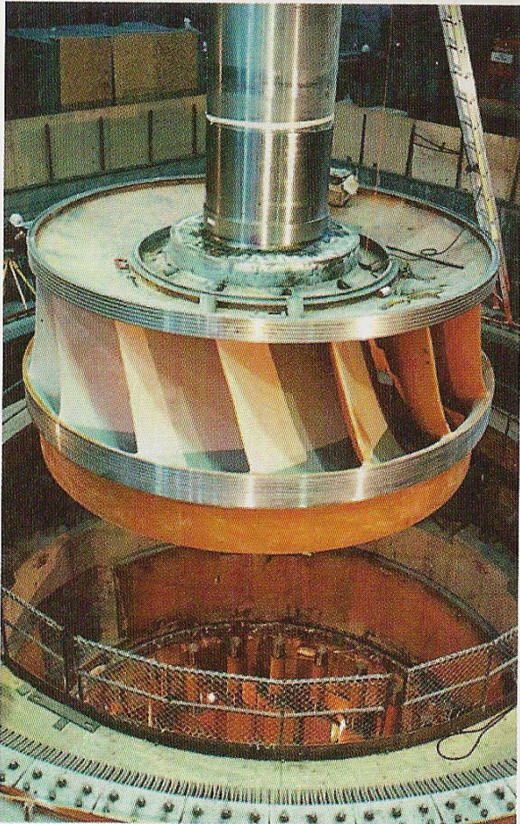
Assemblage d'une turbine à la centrale La Grande-2. Lorsque l'eau la fait tourner, cette turbine actionne un générateur large de plusieurs mètres.
