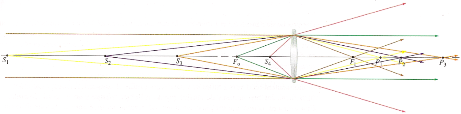
Figure 26.14 Lorsque la source s'approche, les rayons qu'elle émet et qui tombent sur la lentille deviennent de plus en plus divergents et l'image s'éloigne de la lentille. Lorsque l'objet atteint le point focal, les rayons émergents ne convergent plus; ils sont parallèles. Si la source est encore plus proche de la lentille, les rayons émergents deviennent divergents et l'image devient virtuelle.
