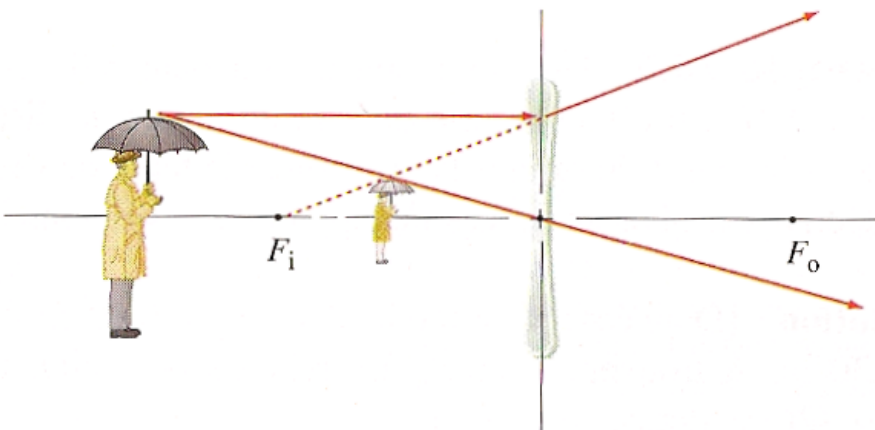
Figure 26.14 Lorsque la source s'approche, les rayons qu'elle émet et qui tombent sur la lentille deviennent de plus en plus divergents et l'image s'éloigne de la lentille. Lorsque l'objet atteint le point focal, les rayons émergents ne convergent plus; ils sont parallèles. Si la source est encore plus proche de la lentille, les rayons émergents deviennent divergents et l'image devient virtuelle.
